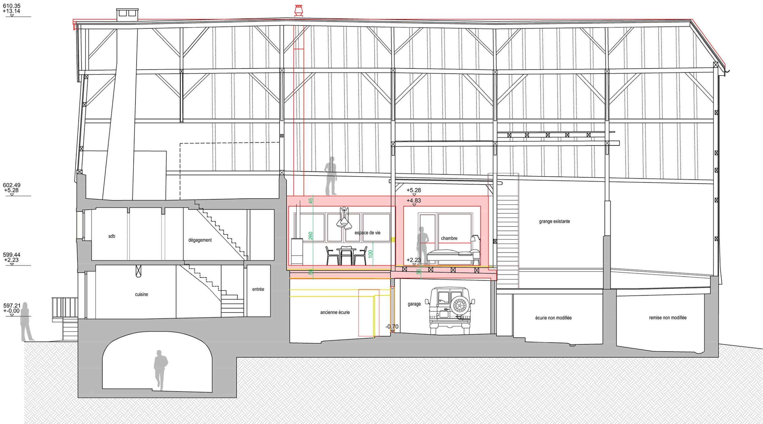
Coupe longitudinale B
