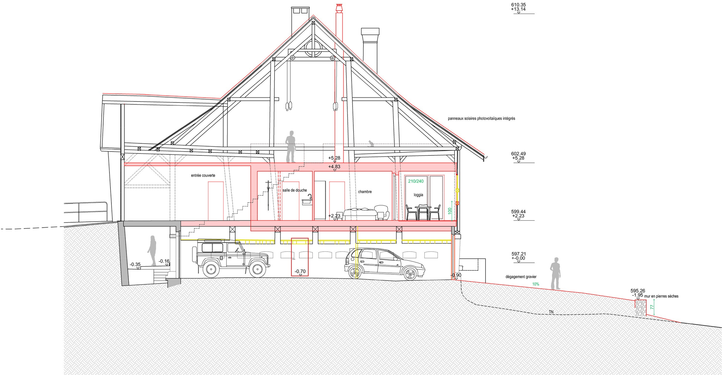
Coupe transversale A
