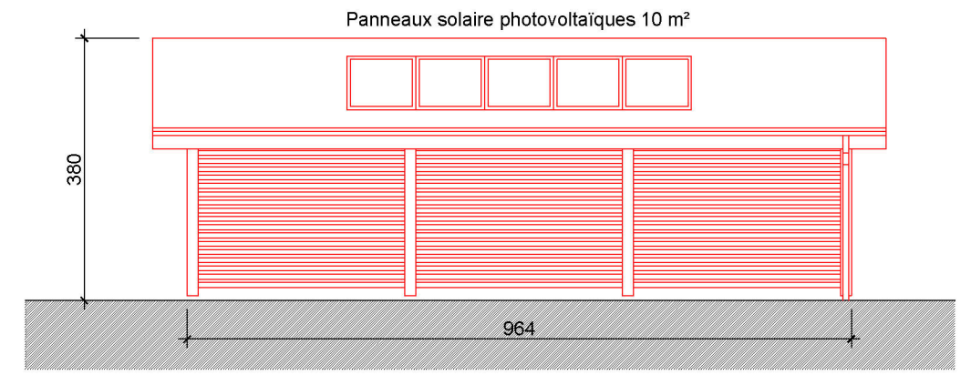
Elevation Sud
