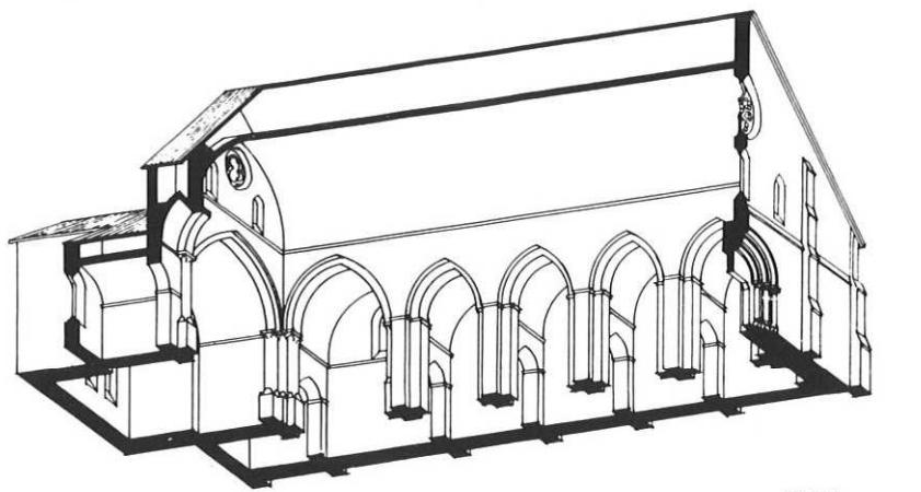
35 PERSPECTIVE ISOMÉTRIQUE DE L'ÉGLISE ABBATIALE DE LA MAIGRAUGE (NEF RECONSTITUÉE)
